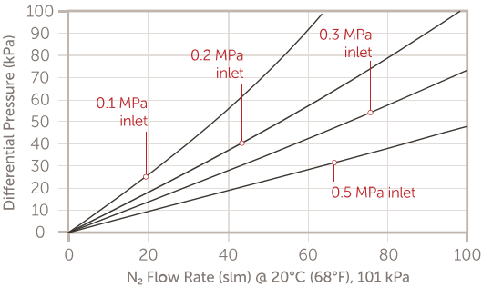
Wafergard III NF Mini XL 1/2" VCR WG3NS2RR4
