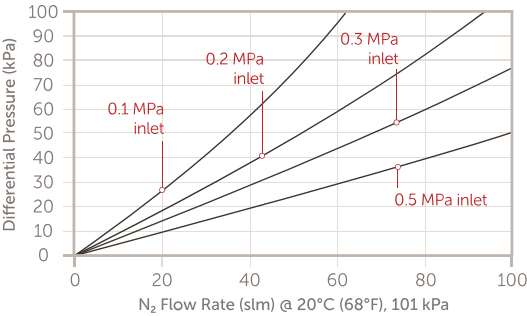
Wafergard III NF Mini XL 1/4" VCR WG3NS2RR2
