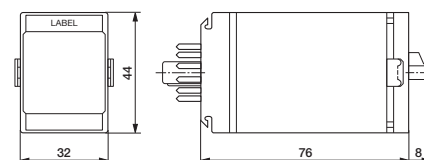
fig. 4. Dimensions (mm)
